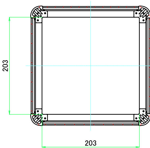
C-C ( 1 : 4.5 )
