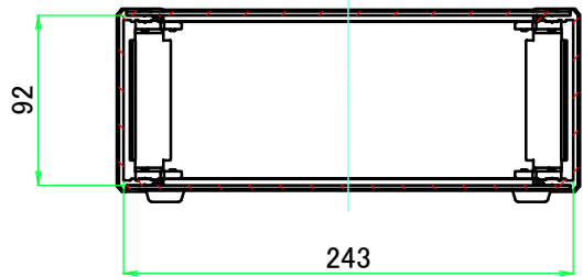
B-B ( 1 : 4.5 )
